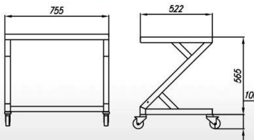
СХЕМА ПОДСТАВКИ
