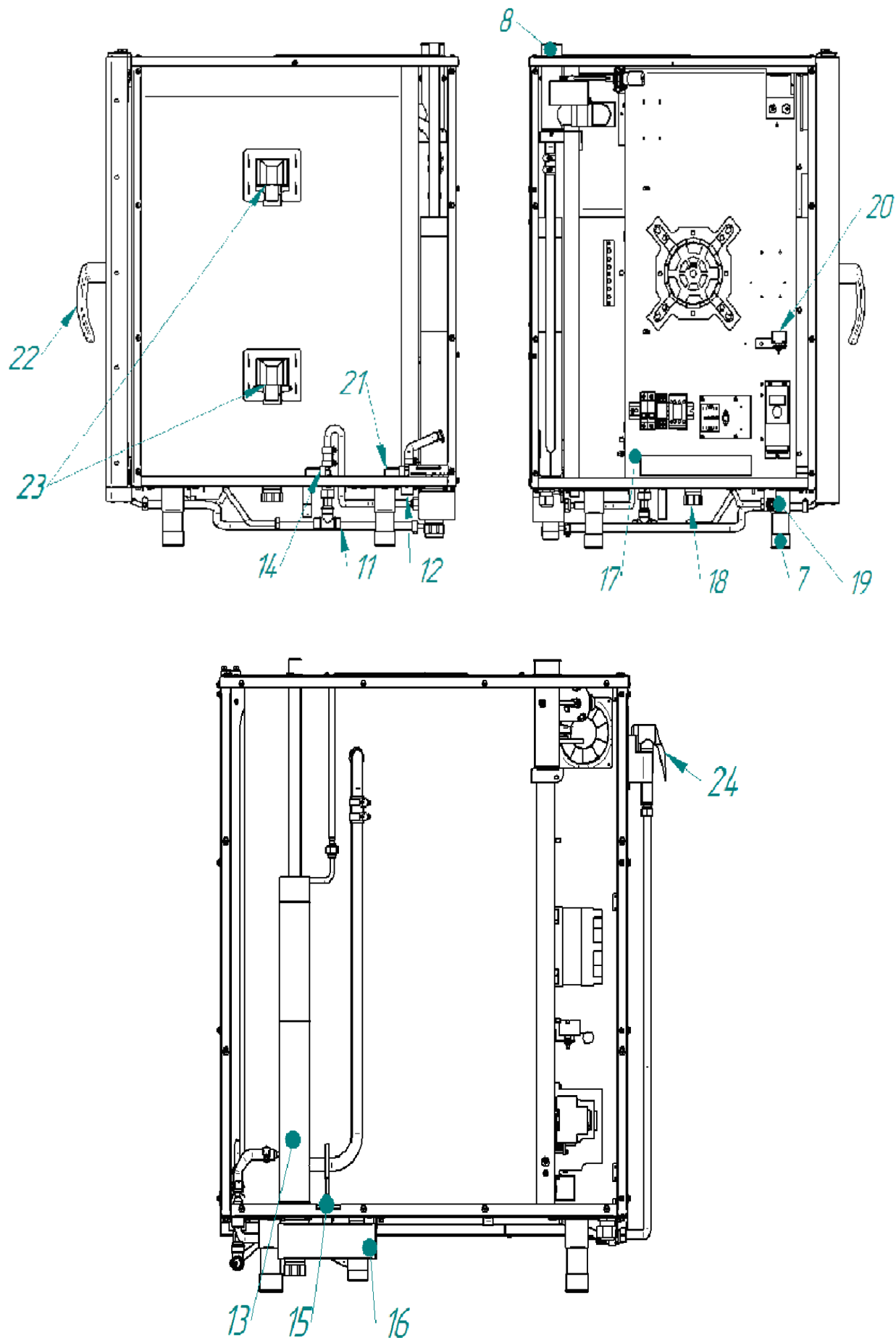
Рис. 1.2 Общий вид пароконвектомата
