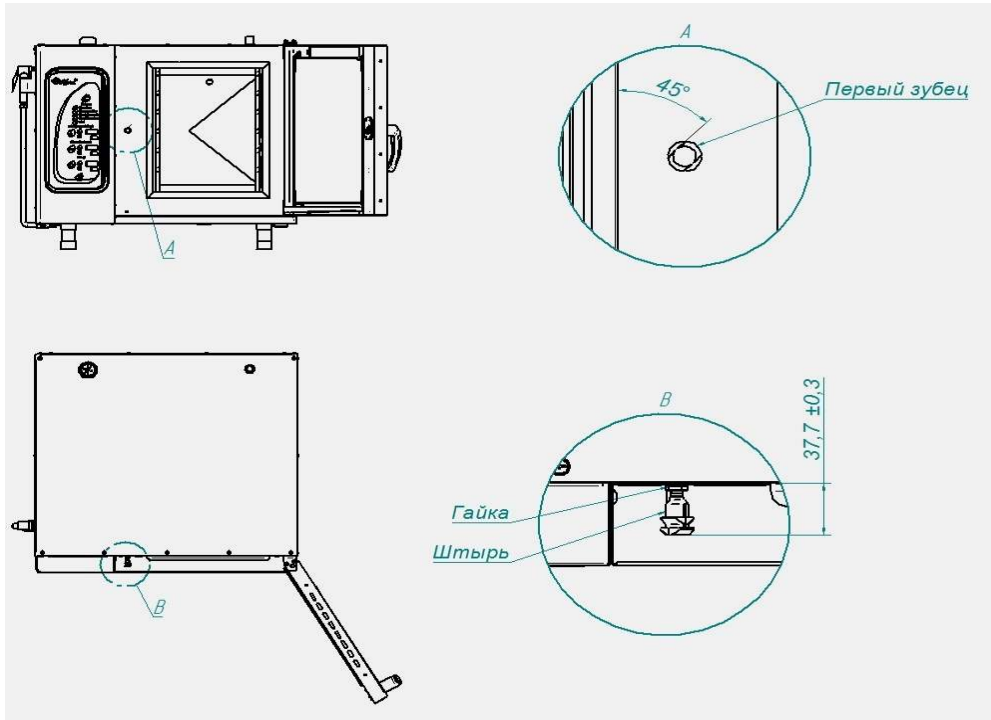
Рис. 10. Регулировка замкового устройства
