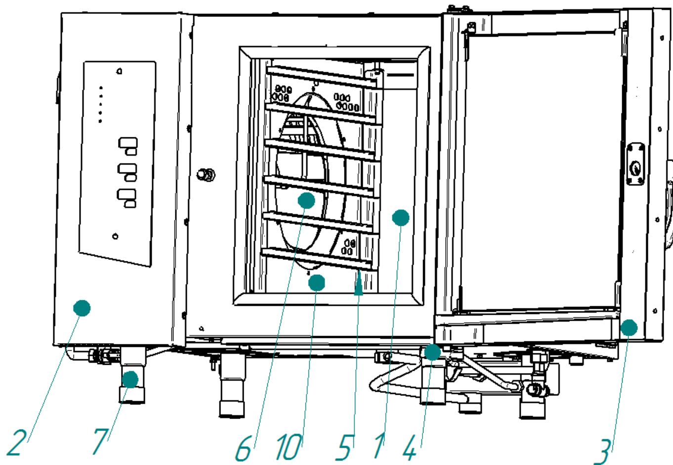
Рис. 1.1 Общий вид пароконвектомата
