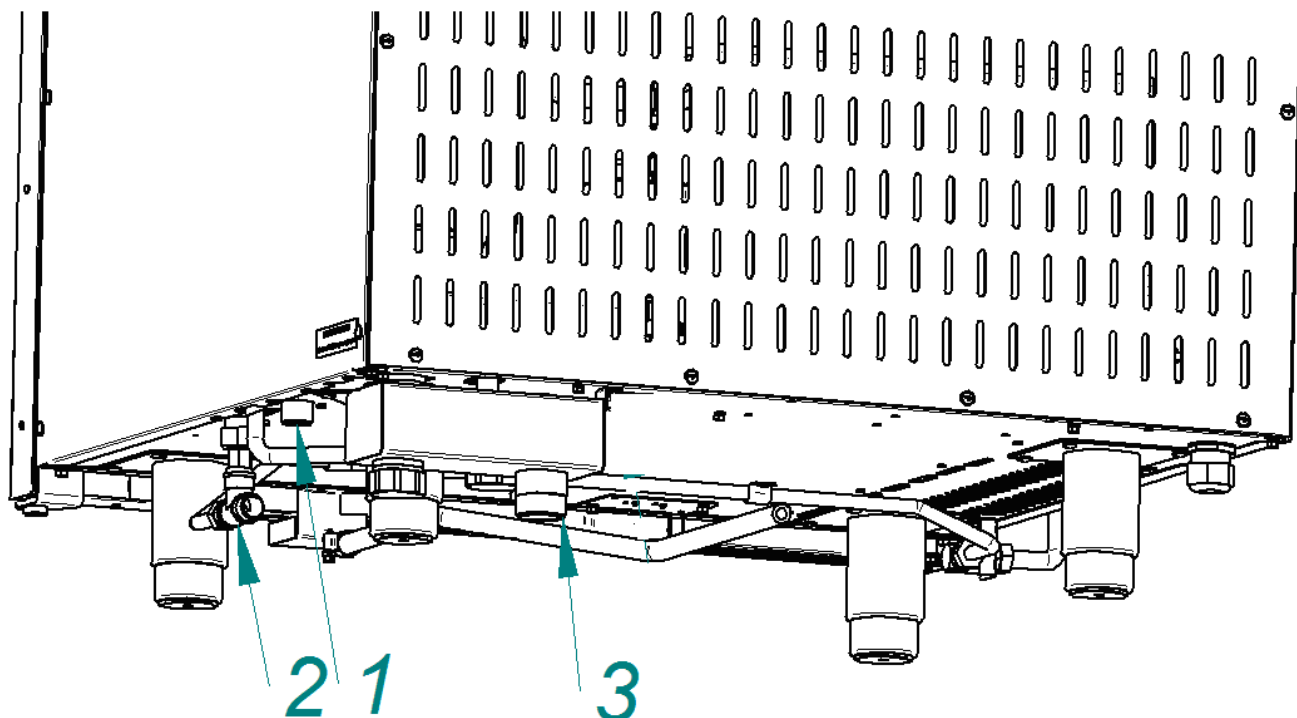
Рис. 4. Подключение к системе водоснабжения
