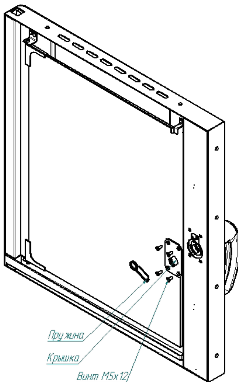
Рис. 9. Ремонт замкового устройства
