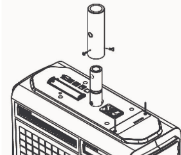
Рисунок 1.11 – Порядок монтажа верхних кронштейнов
