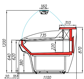
НИЗКОТЕМПЕРАТУРНАЯ
