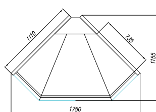
ВНЕШНИЙ УГОЛ
