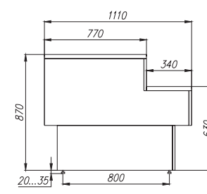
НЕЙТРАЛЬНЫЙ ПРИЛAVOK
