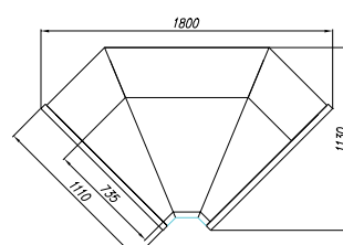
ВНУТРЕННИЙ УГОЛ
